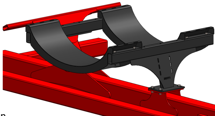
Step 3 - 500 Gallon
